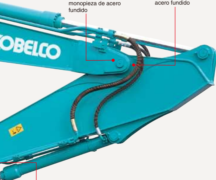
Base del brazo de acero fundido
